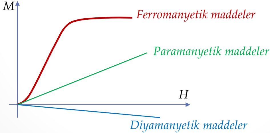
Ferromanyetik madde
